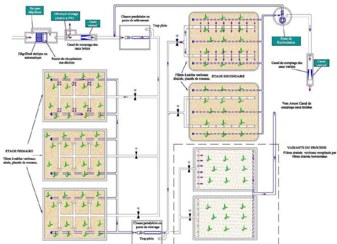
Figure 3 : Vue en plan d'une STEU type « filtre planté de roseaux à deux étages » (Source : Les procédés d'épuration des petites collectivités Agence de l'Eau Rhin Meuse)
