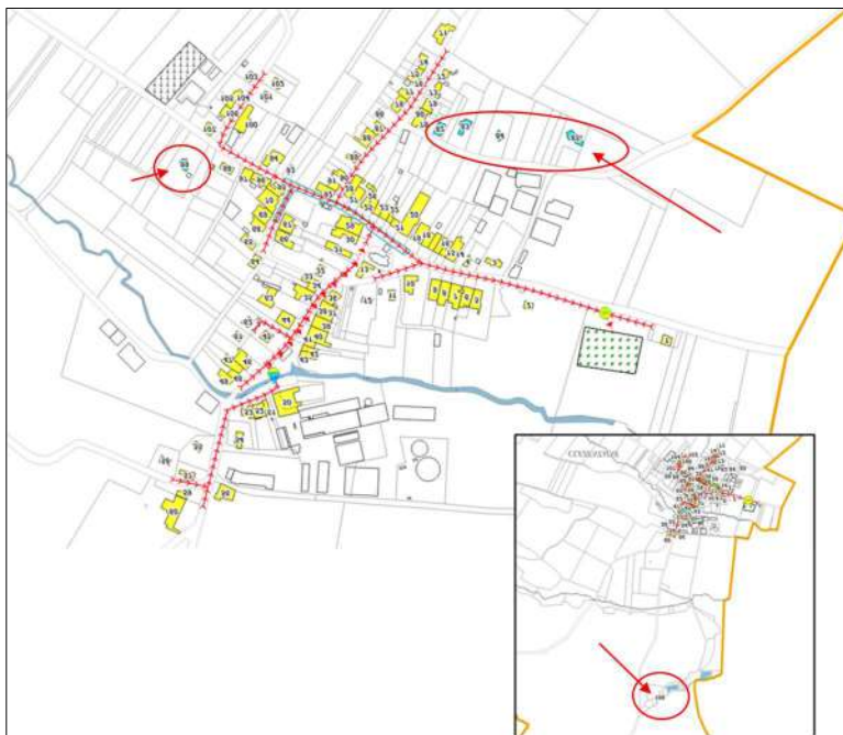
Figure 6 : Immeubles concernés par le zonage ANC dans le scénario 2
