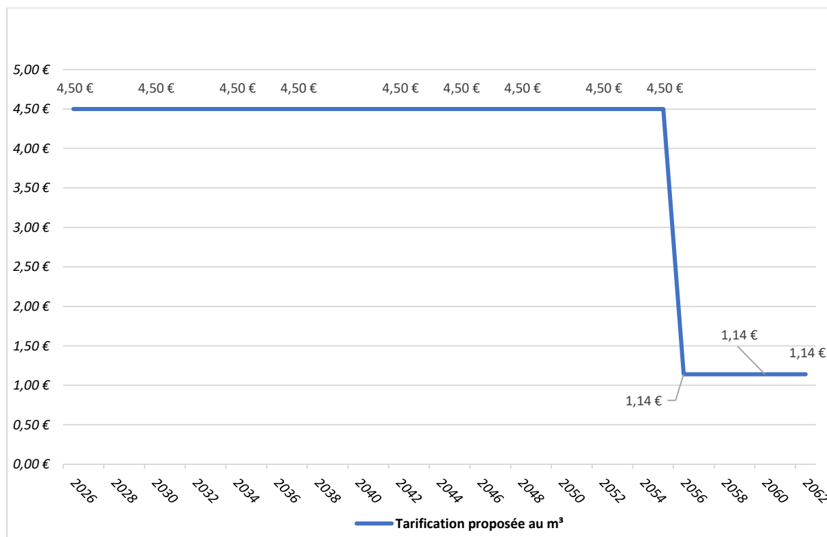
Figure 15 : Proposition du prix de l'assainissement en €/m³ – simulation à 30% d'aides (sc 3)
