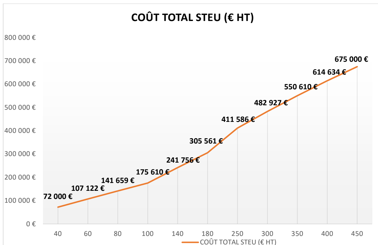
Figure 6 : Evolution du coût d'une STEU en fonction de sa capacité de traitement exprimée en EH
