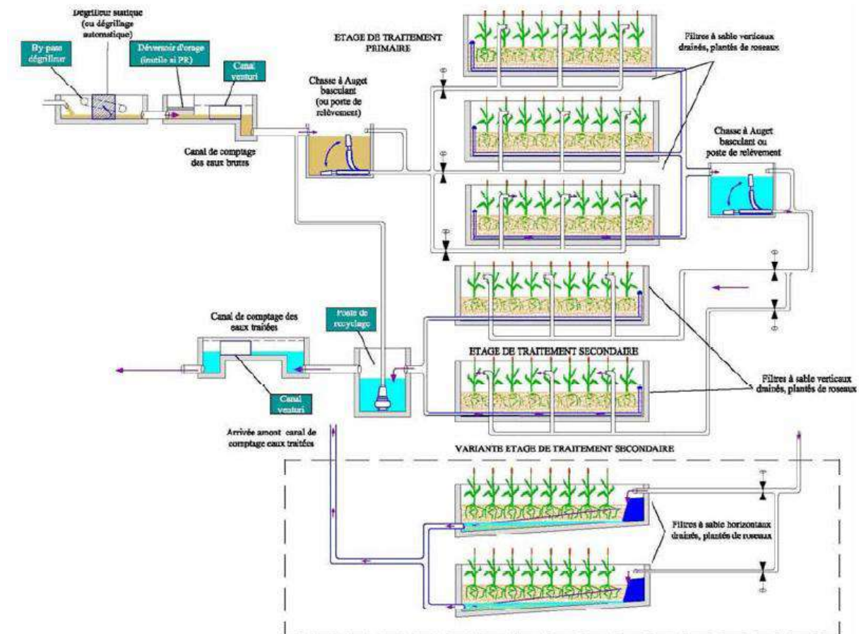
Figure 3 : Vue en coupe d'une STEU de type « filtre planté de roseaux à deux étages » (Source : Les procédés d'épuration des petites collectivités Agence de l'Eau Rhin Meuse)
