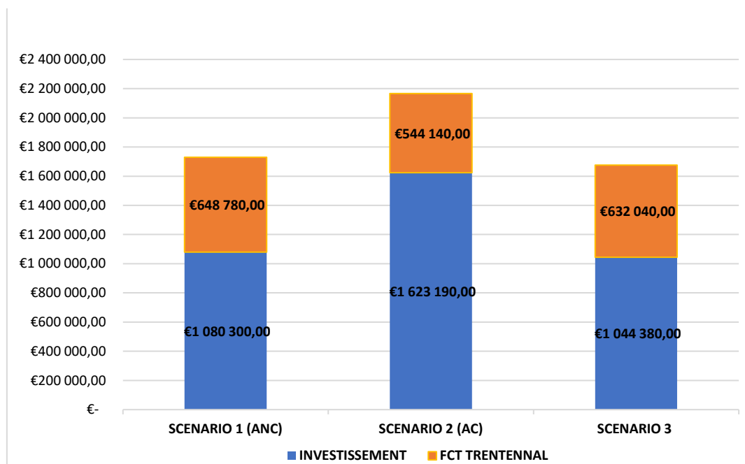
Figure 8 : Comparatif des coûts liés aux scénarios d'assainissement
