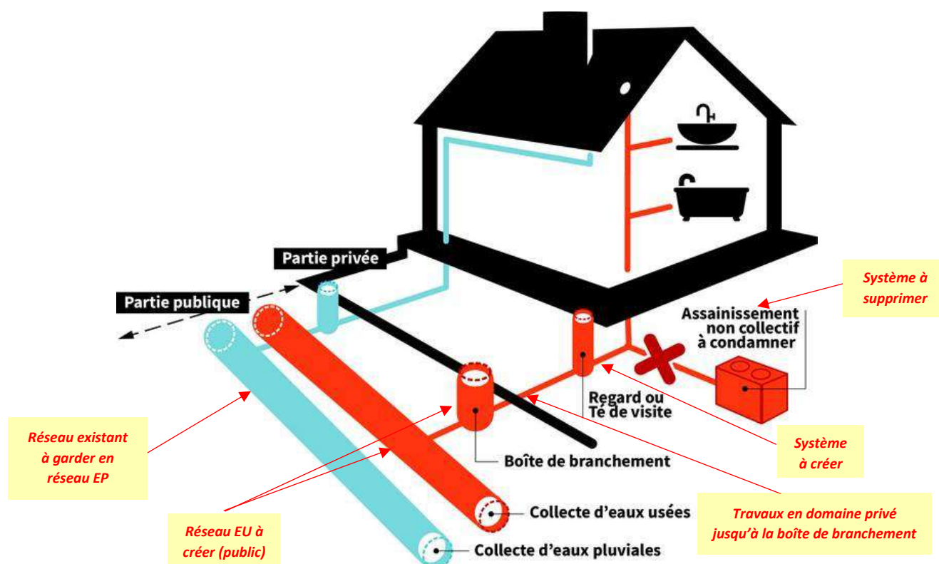
Figure 5 : Système de collecte pour l'assainissement collectif (source : CC Haut Val de Sèvre)
