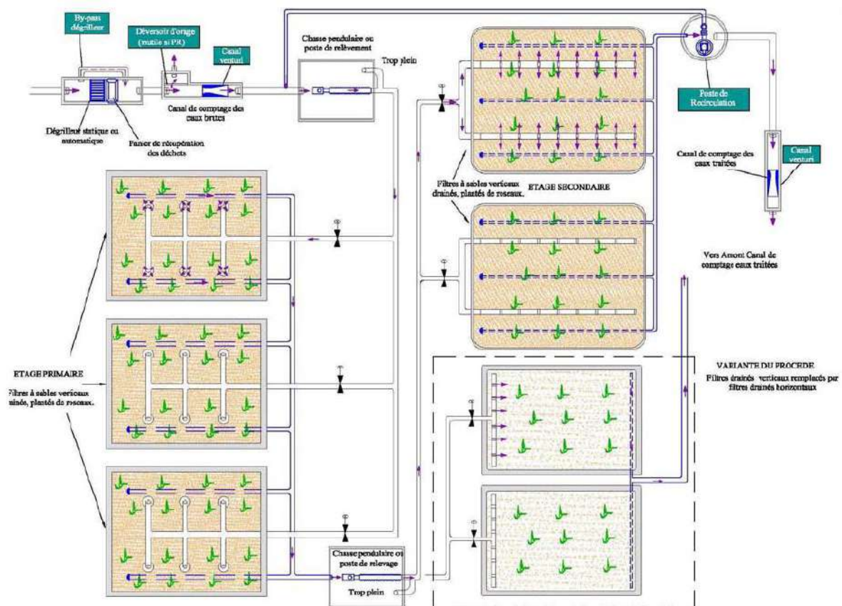
Figure 4 : Vue en plan d'une STEU type « filtre planté de roseaux à deux étages » (Source : Les procédés d'épuration des petites collectivités Agence de l'Eau Rhin Meuse)
