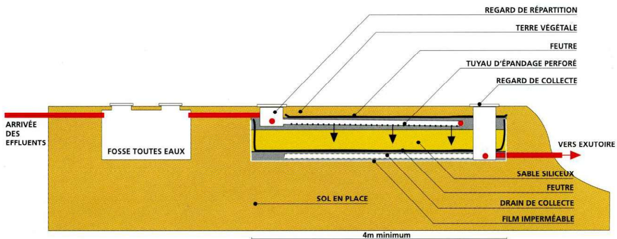
COUPE LONGITUDINALE
