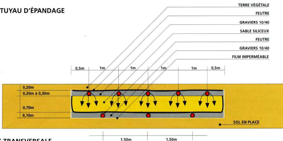
COUPE TRANSVERSALE
