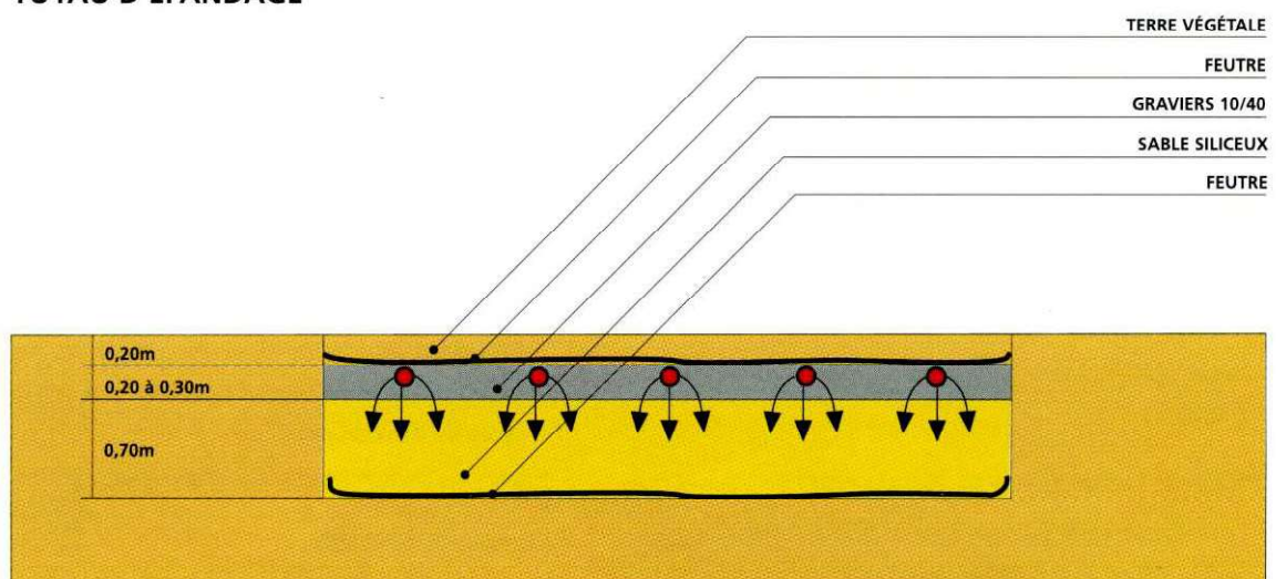
TUYAU D'ÉPANDAGE
