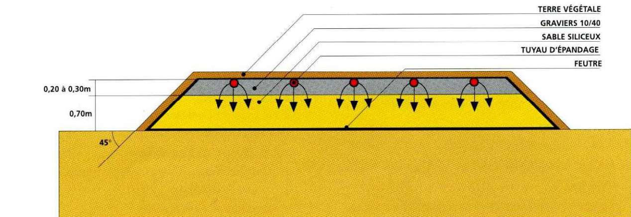
COUPE TRANSVERSALE
