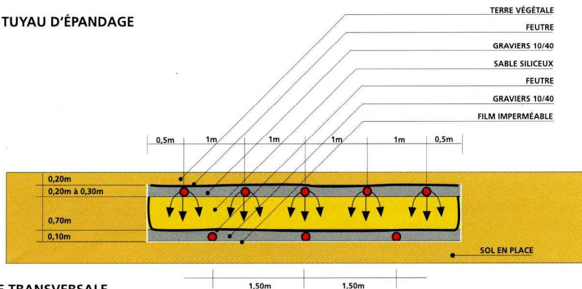
COUPE TRANSVERSALE
