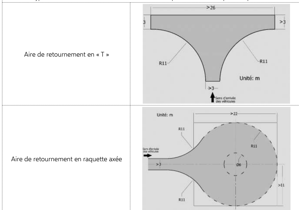
Schéma type de dimensionnement des aires de retournement pour les voies en impasse de plus de 50 mètres
