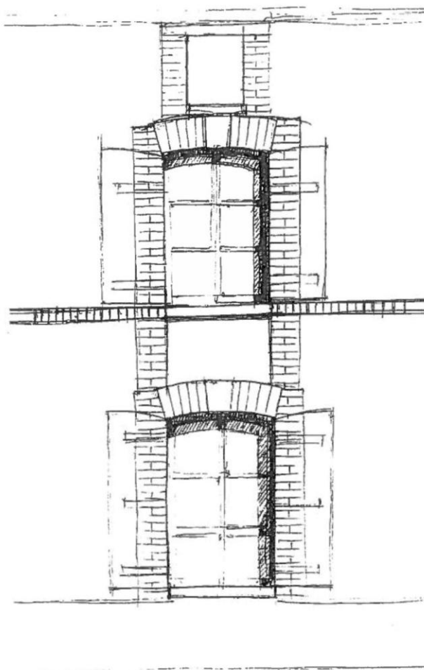
Fenêtres en travée. Appareillage de briques et pierres en clefs et en appuis. Milieu du XIXe siècle
