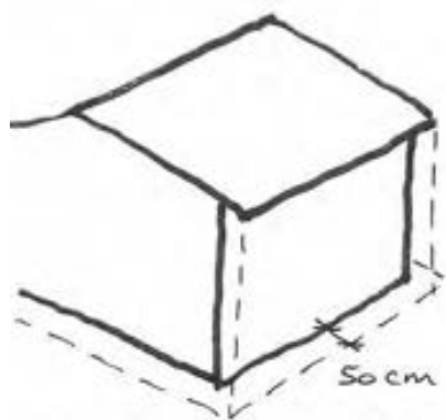
Projection des débords de toiture : 50 cm maximum
