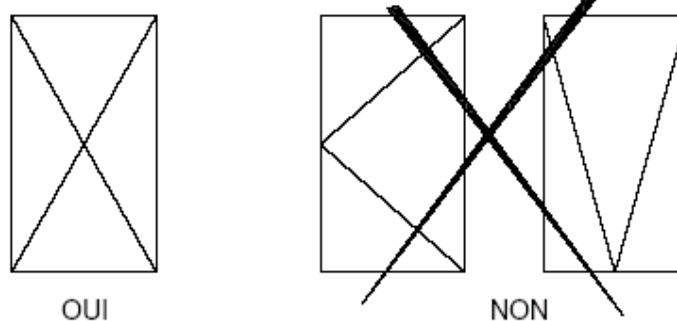
Principe de contreventement
