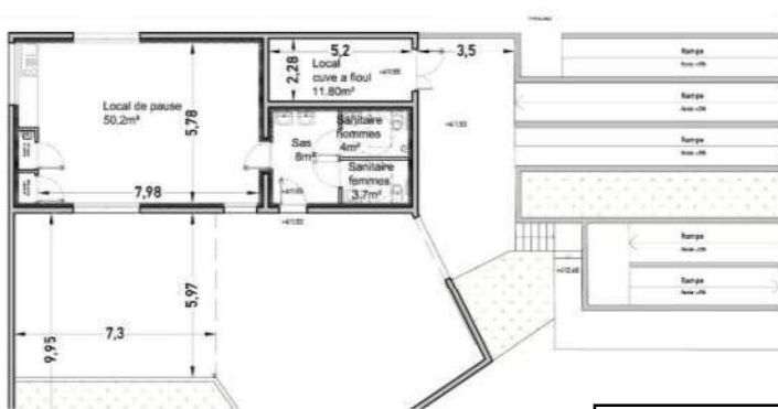
Plan RDC
