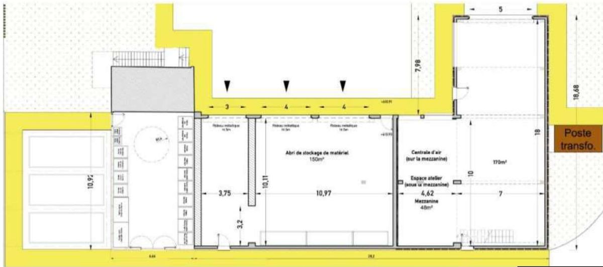
Plan RDC
