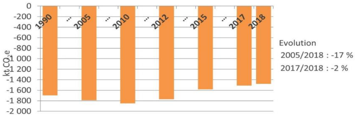
Illustration n°14. Evolution des flux de carbone entre l'atmosphère et le secteur UTCATF (PRG 2013) source Atmo Grand Est, Invent'air V2020
