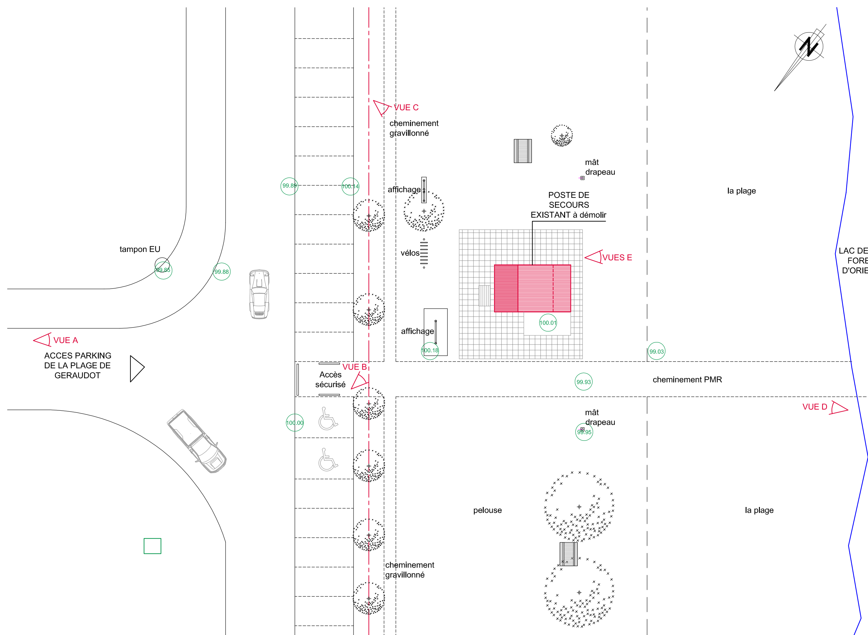
PLAN DE MASSE- ETAT EXISTANT - Ech 1/200° - SEPTEMBRE 2021
