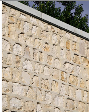
Interprétation contemporaine du mur moellons de pierre calcaire, construction en "pierre banchée" Angoulême (16), A. Chemetoff architecte photo Ph. Peyrefitte arch.
